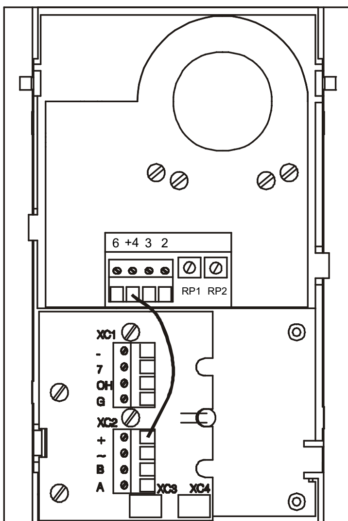
Pohľad na svorkovnice Pohľad na svorkovnice
