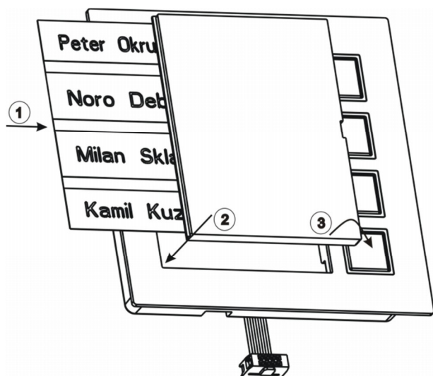
Obr.27 vkladanie menoviek do modulov Tx
