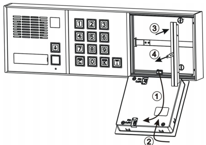
Obr.19 Horizontálna zostava VEV+TM13+info
