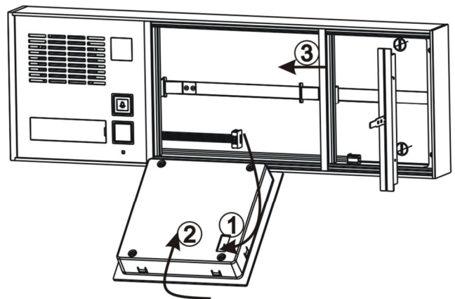
Obr.17 Montáž tlačidlového modulu
