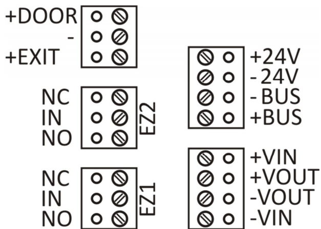
Obr.29 Význam - elektrické priradenie svoriek svorkovnic modulov EV/VEV
