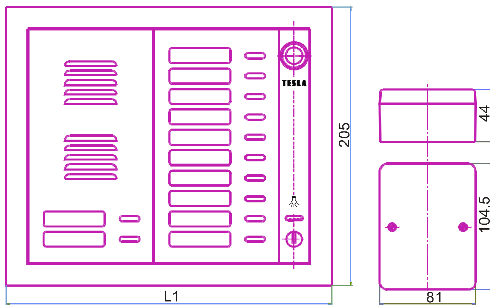
Obr.1 Tlačidlové tablo 4 FP 831 .../1KS1
