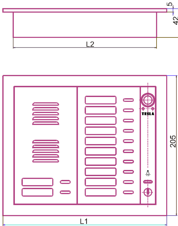
Obr.3 Tlačidlové tablo 4 FP 831 .../2KS1
