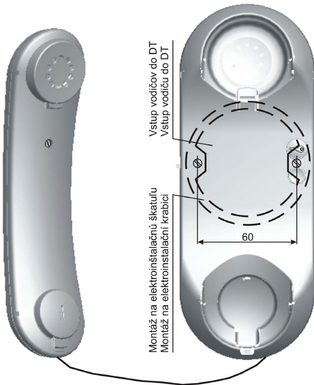
obr.3 Montáž DT ESO na elektroinštalačnú škatuľu Montáž DT ESO na elektroinštalačnej krabici
